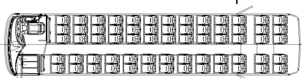
65座位平面圖
